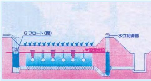
地下水制御システム図
