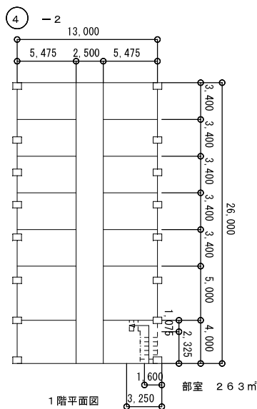
1階平面図
