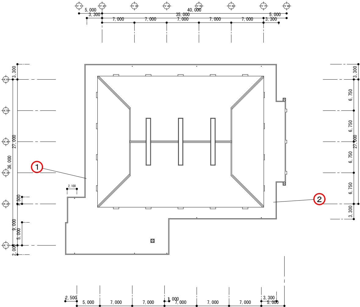
R 階平面図
