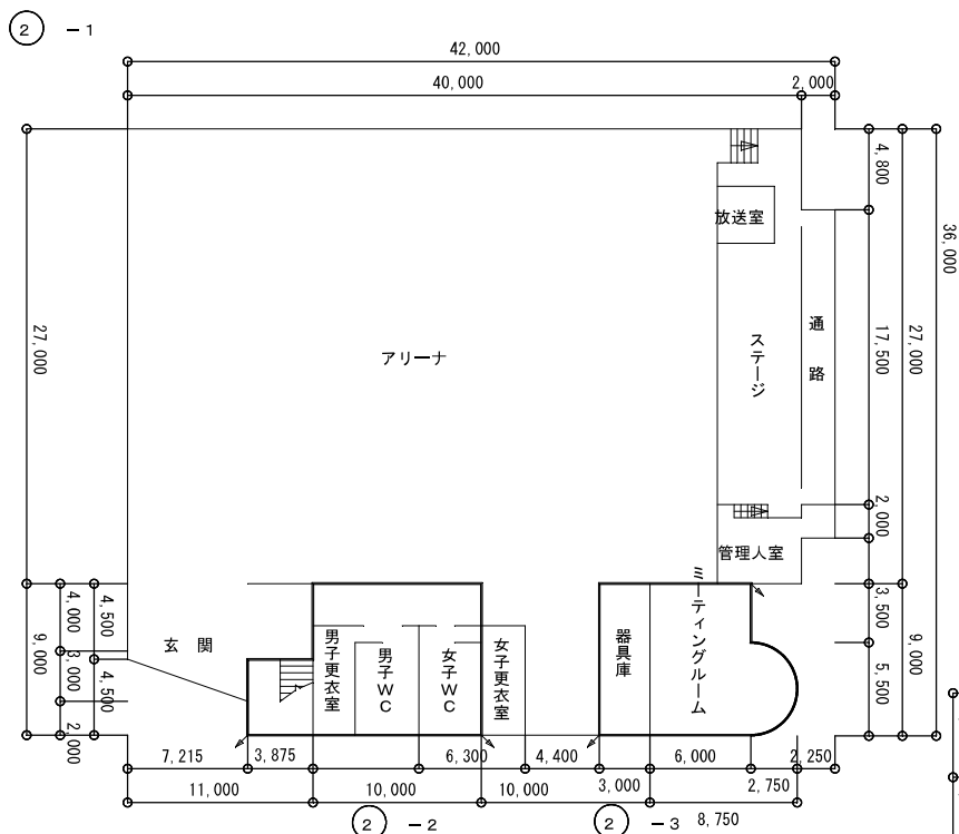
1階平面図
