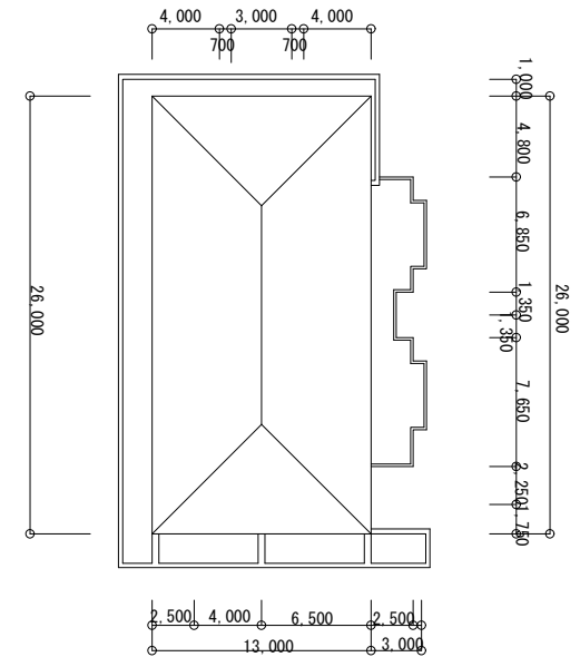
R 階平面図
