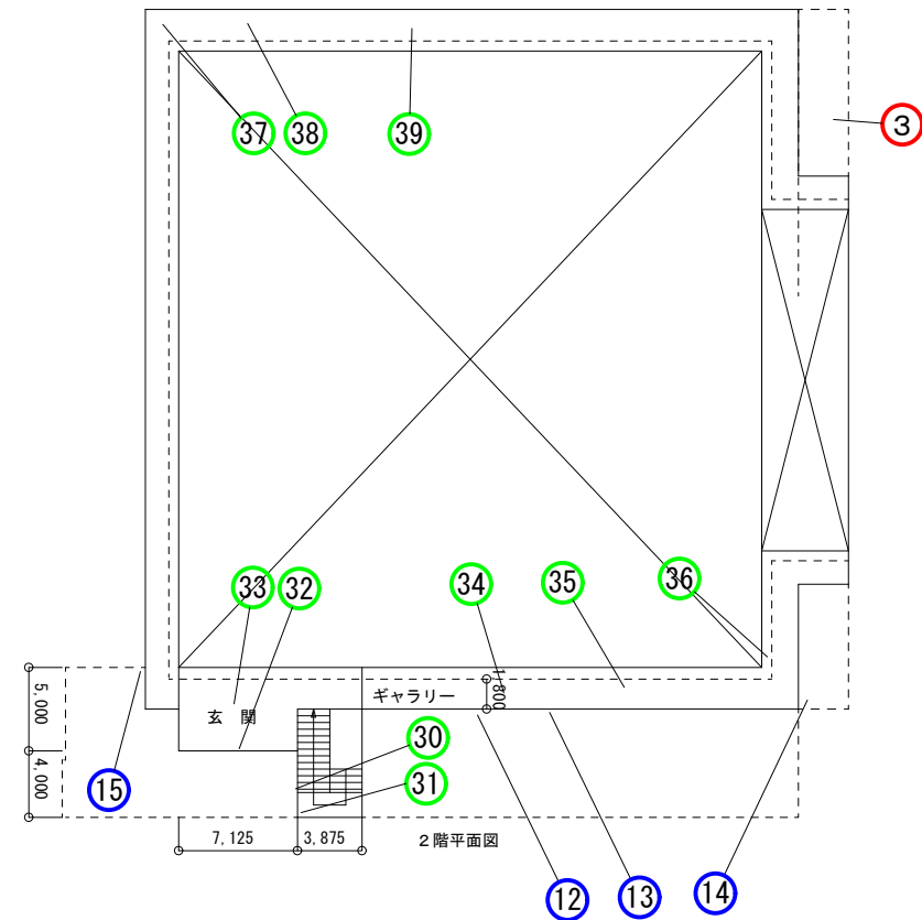
2 階平面図
